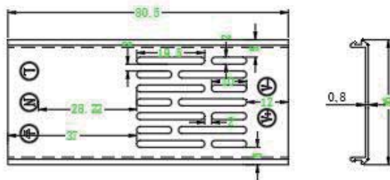
KHT系列30W 上盖 上盖激光割孔 打字不用管
